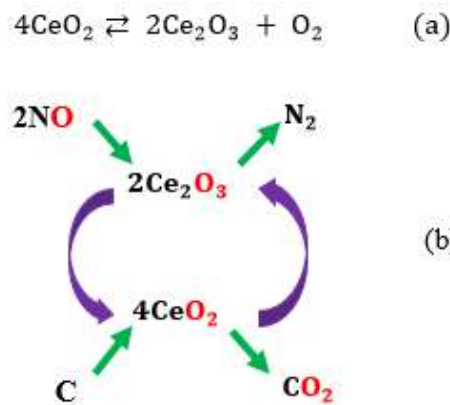
Şekil 3. (a) CeO 2 tersinir oksijen salınımı, (b) yanma sürecindeki katalizör görevi
