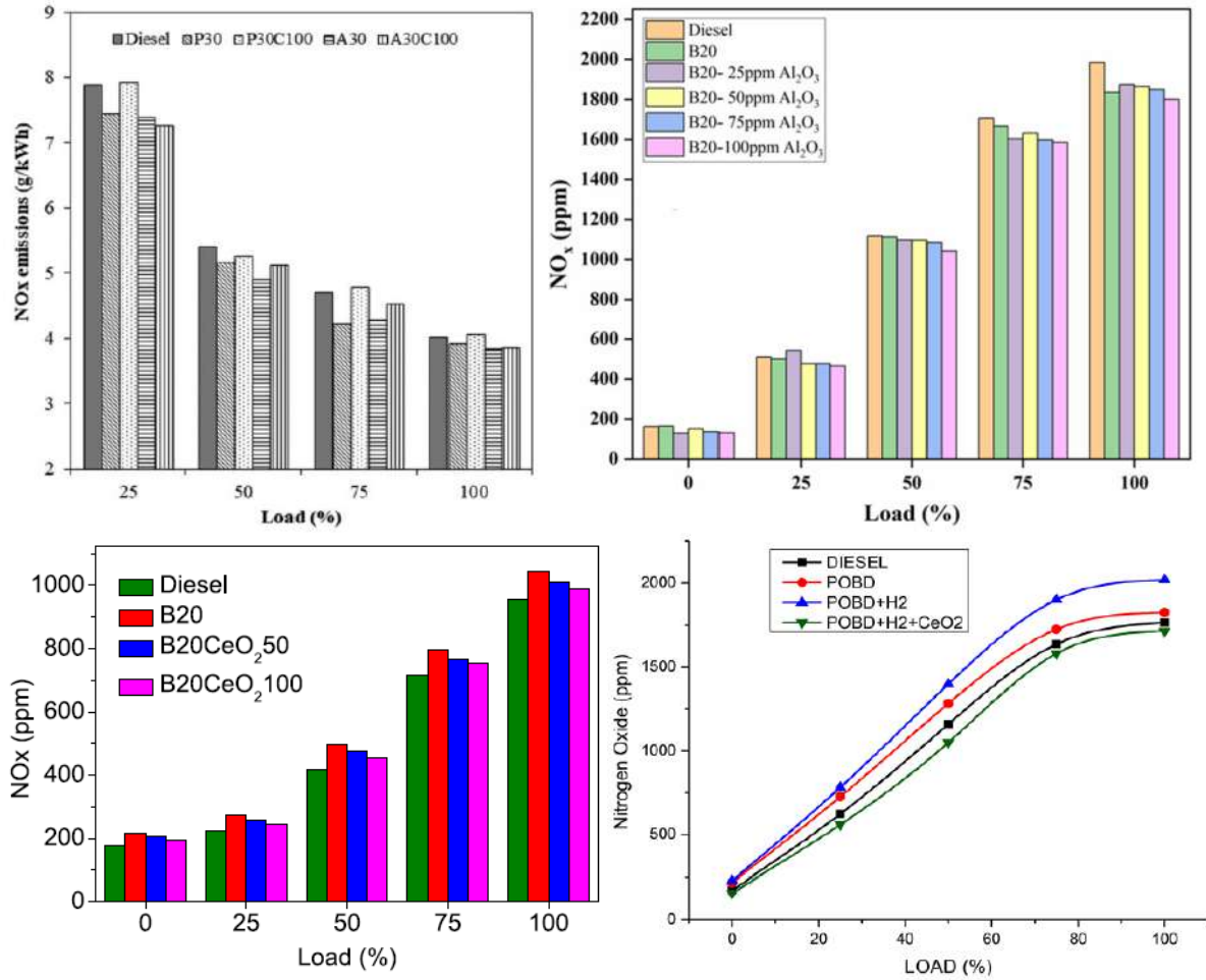
Şekil 8. NOx emisyonunun motor yüküne bağlı değişimi[3,5,23,24]
