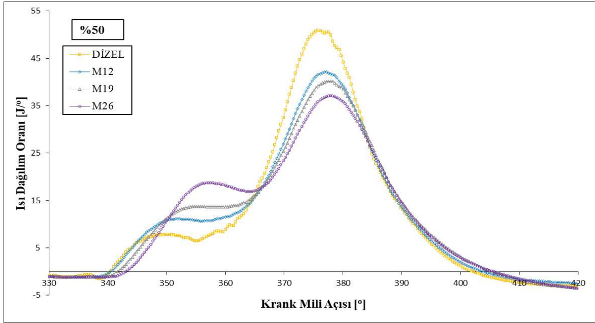
Şekil 8. %50 kısmi yükte dizel, M12, M19 ve M26 yakıtları için oluşan ısı dağılım oranları
