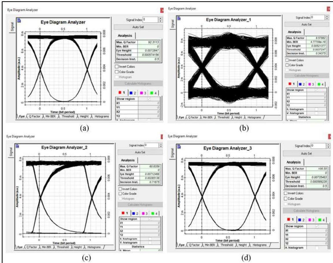
Şekil 7. (a) Gaussian optik filtre, (b) Dikdörtgen optik filtre, (c) Butterworth optik filtre ve (d) Bessel optik filtre için göz diyagramları
