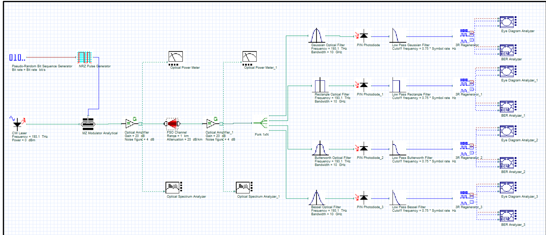
Şekil 3. Optik filtrelerin eklendiği sistem
