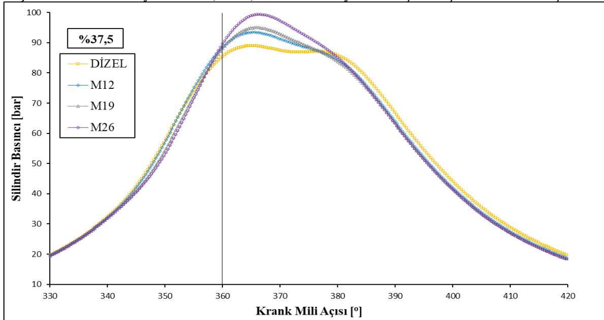
Şekil 3. %37,5 kısmi yükte dizel, M12, M19 ve M26 yakıtları için oluşan silindir basınçları
