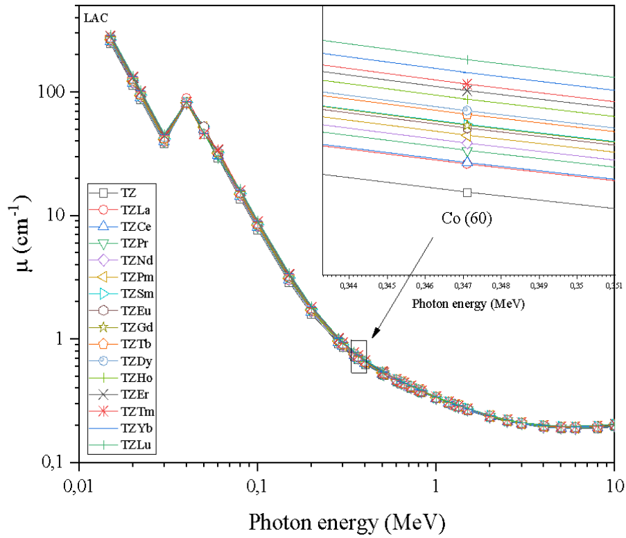
Şekil 2. Numunelere ait ( \mu ) ~ foton enerjisi (photon energy) (LAC) grafiği
