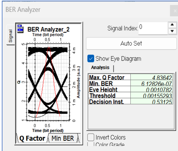
c) 10 Gbps, 1500 m ve 8 kullanıcı
