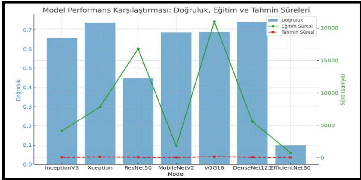
Şekil 1: Modellerin Doğruluk, Eğitim ve Tahmin Süreleri Grafikleri
