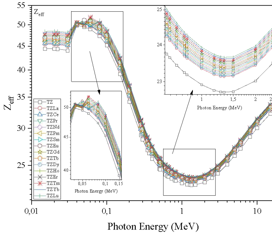
Şekil 5. Numunelere ait etkin atom numarası ~ foton enerjisi (photon energy) ( Z_{eff} ) grafiği
