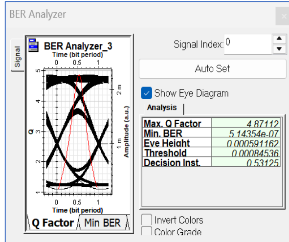
d) 10 Gbps, 1500m ve 16 kullanıcı
