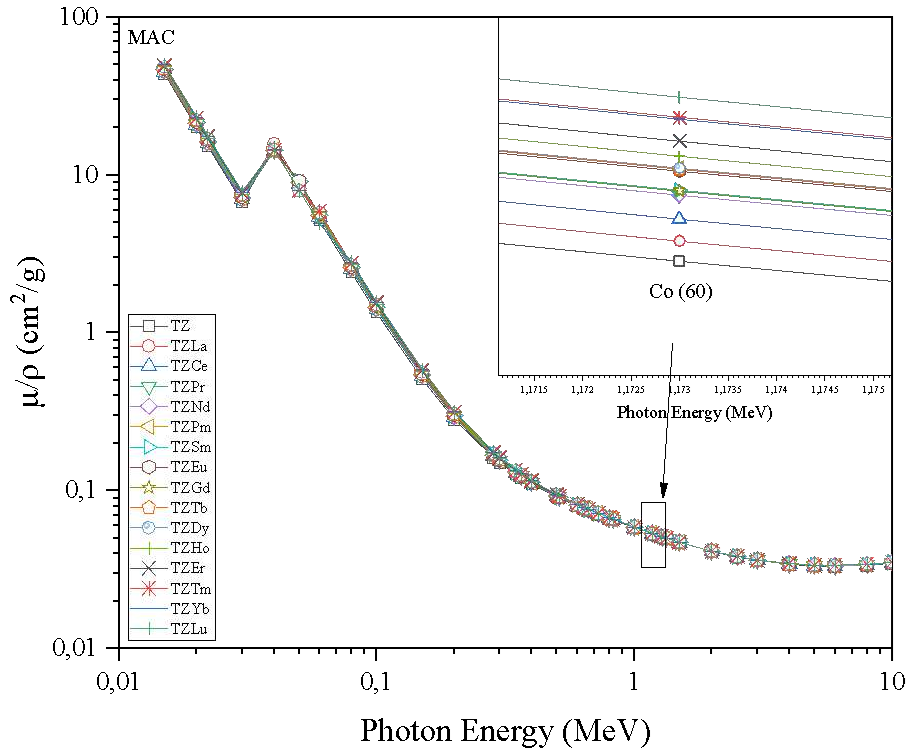
Şekil 1. Numunelere ait (\mu/\rho) \sim foton enerjisi (photon energy) (MAC) grafiği
