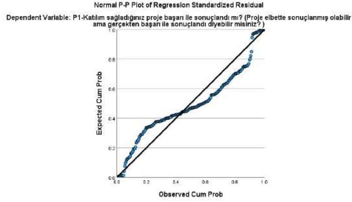
Şekil 4. Normal P-P Grafiği
