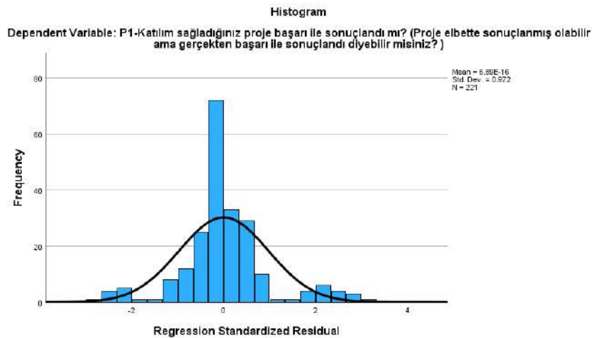
Şekil 3. Histogram
