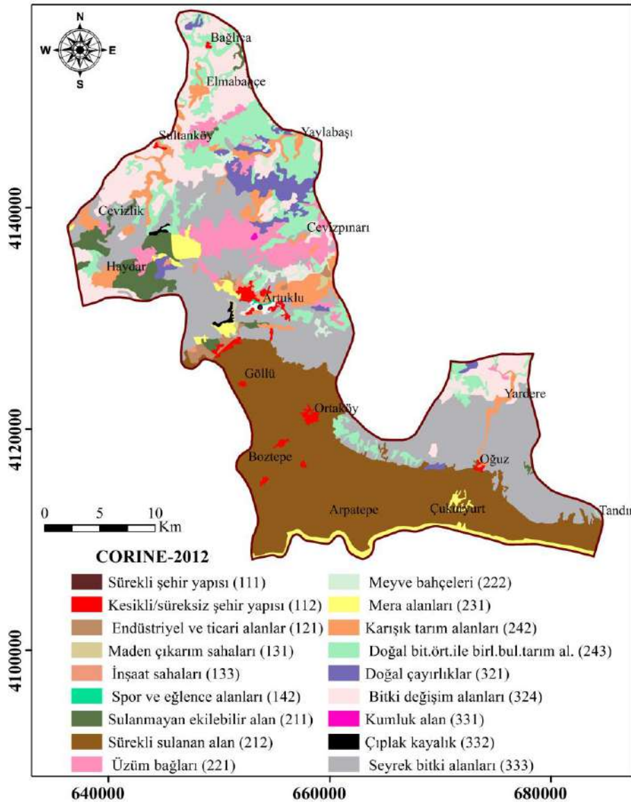
Şekil 6. 2012 yılına ait CORINE arazi örtüsü/kullanımı haritası
