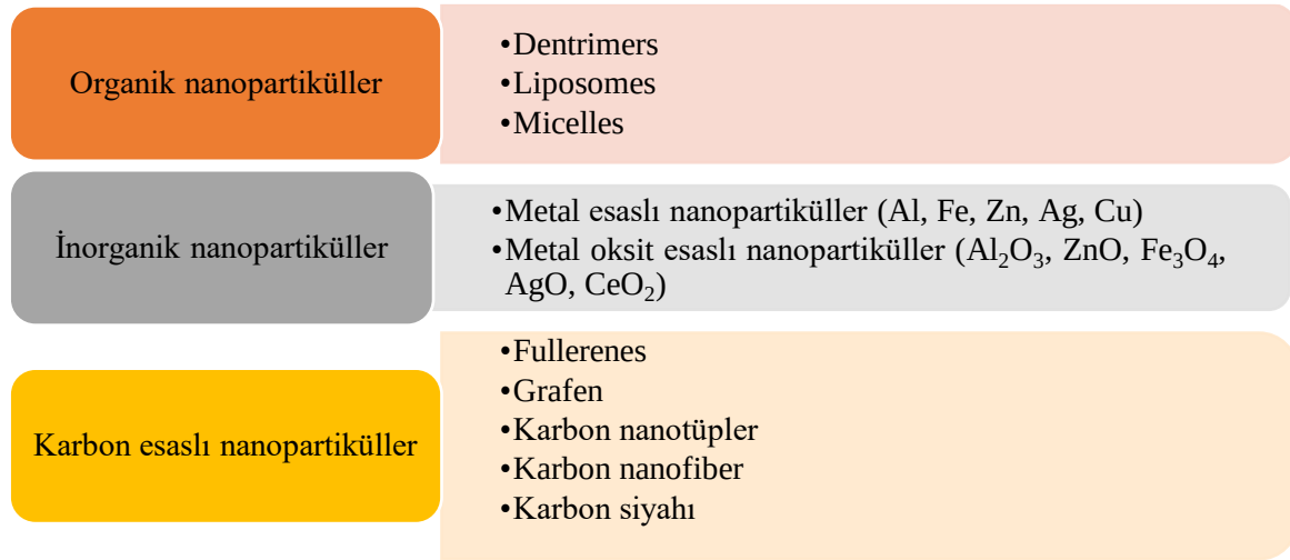
Şekil 2. Nanopartikül türleri
