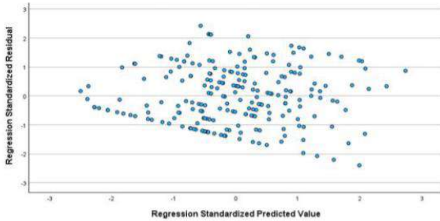
Şekil 5. Saçılım Grafiği
