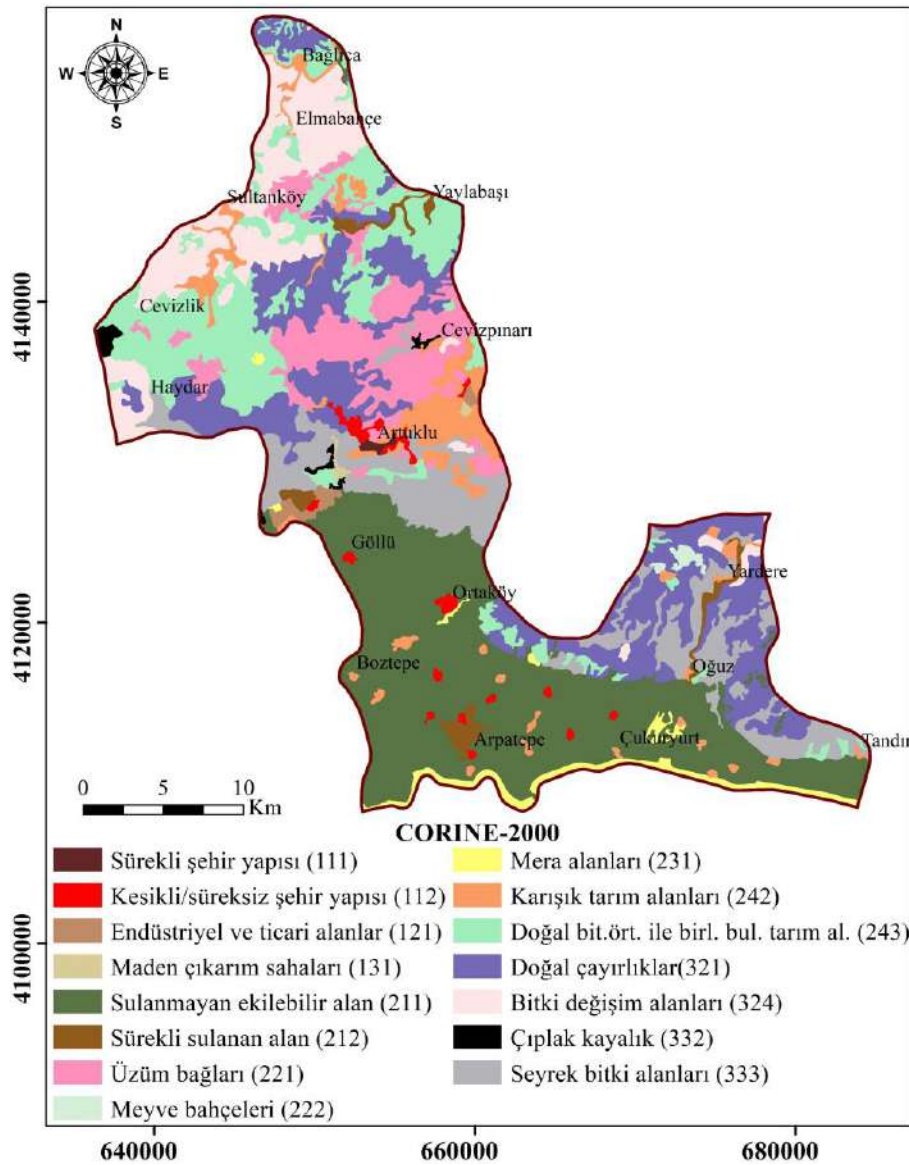
Şekil 4. 2000 yılına ait CORINE arazi örtüsü/kullanımı haritası
