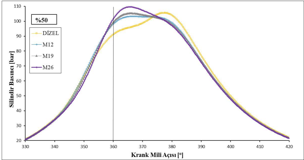
Şekil 4. %50 kısmi yükte dizel, M12, M19 ve M26 yakıtları için oluşan silindir basınçları
