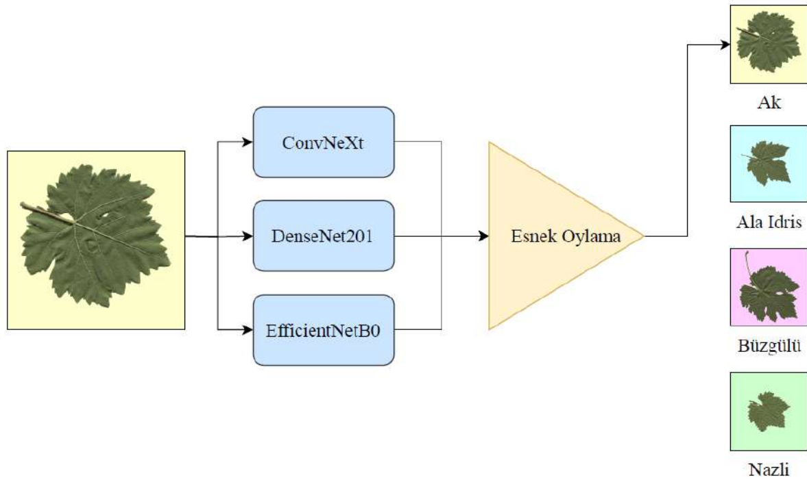
Şekil 2. Önerilen Topluluk öğrenme tabanlı derin sinir ağı ile asma yaprağının sınıflandırmasına ait blok diyagram
