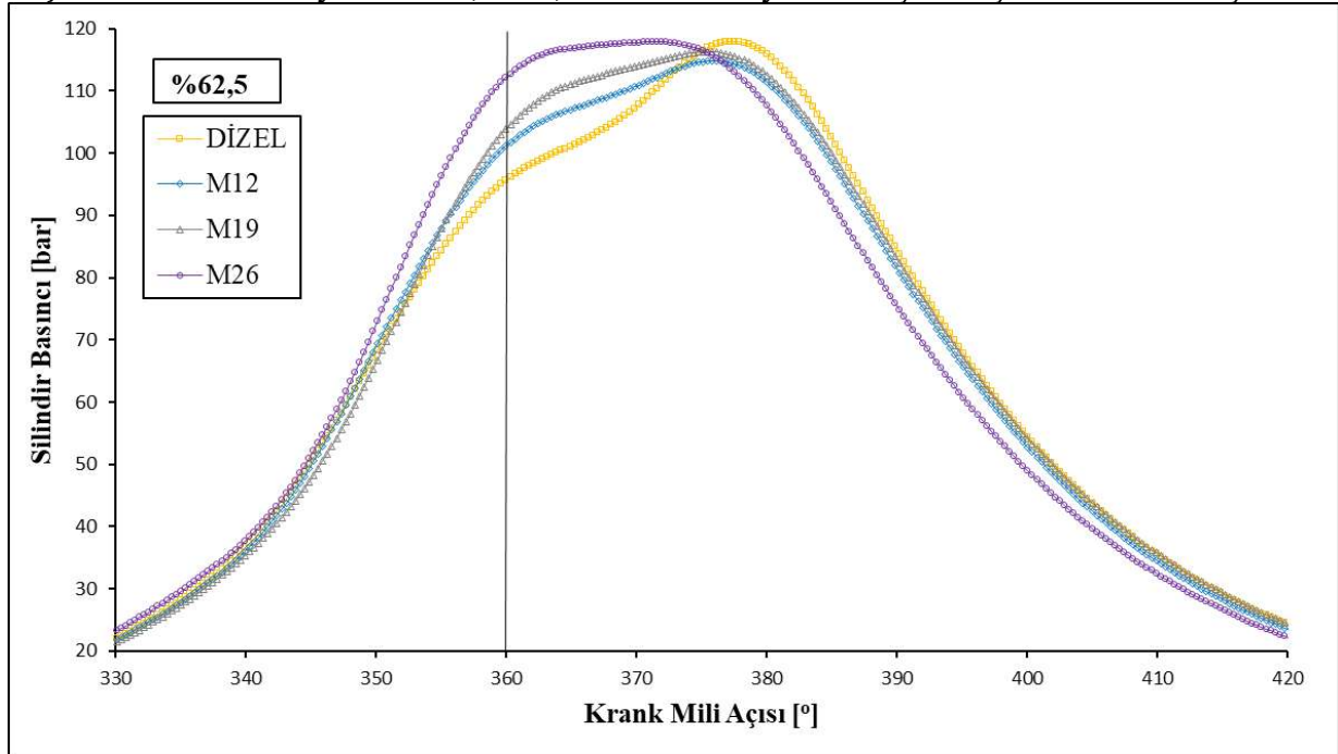
Şekil 5. %62,5 kısmi yükte dizel, M12, M19 ve M26 yakıtları için oluşan silindir basınçları
