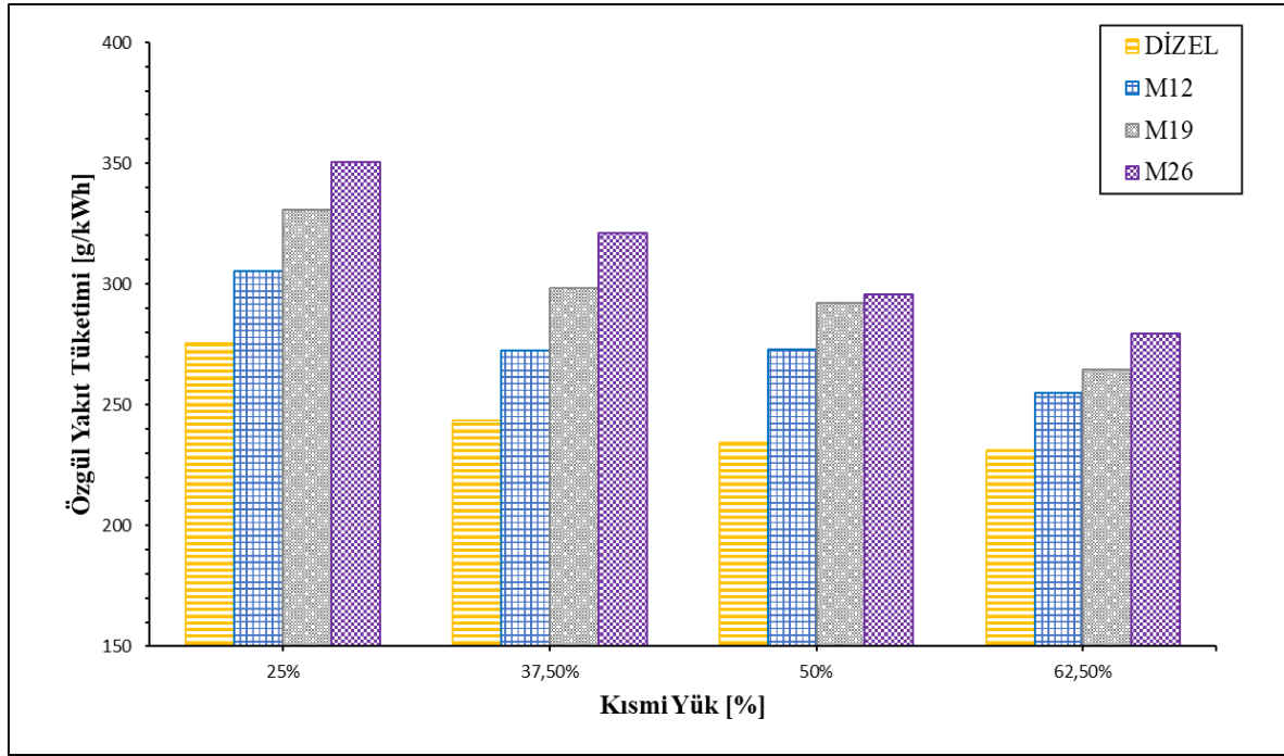
Şekil 10. Farklı kısmi yüklerde meydana gelen özgül yakıt tüketimi değişimleri
