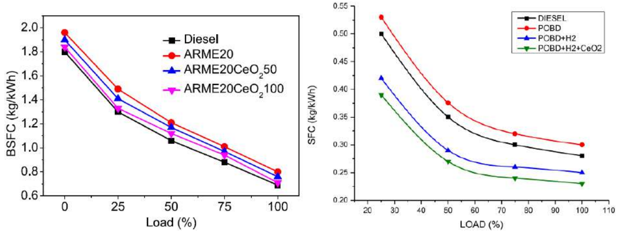
Şekil 5. Motor yüküne bağlı BSFC'nin değişimi [3,5,23,24]
