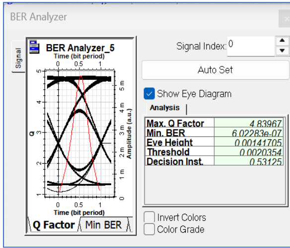
a) 10 Gbps, 600 m ve 8 kullanıcı
