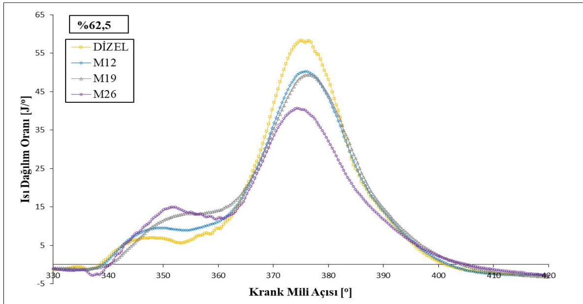
Şekil 9. %62,5 kısmi yükte dizel, M12, M19 ve M26 yakıtları için oluşan ısı dağılım oranları
