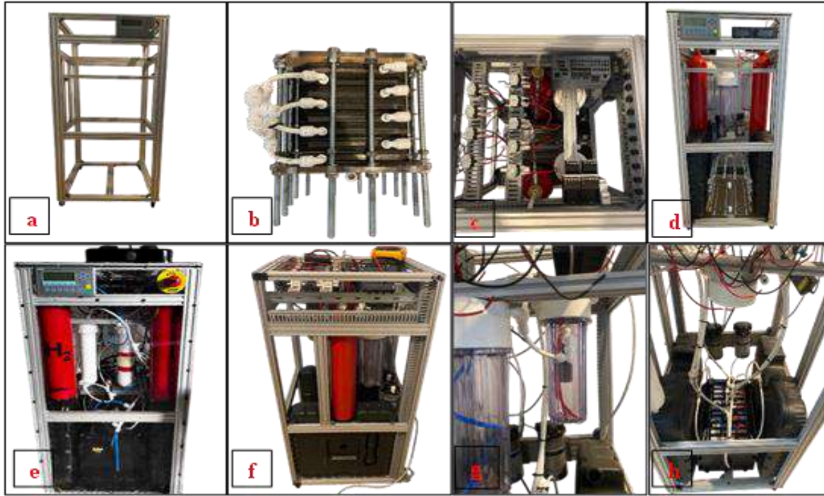
Şekil 2. Cihazın Tasarım Aşamaları - (a) İskelet yapısı oluşumu; (b) Hidrojen reaktörü tasarımı; (c) Valflerin yerleşim düzeni; (d) Atık ve elektrolize olmuş su depoları; (e) Yanma ünitesi dizaynı; (f) Elektriksel bağlantıların kontrolü; (g) Üretilen hidrojenin filtreleme membranlarına aktarımı; (h) Sirkülasyon pompaları ve hortum bağlantıları.
