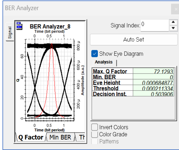
d) 5 Gbps, 600 m ve 64 kullanıcı
