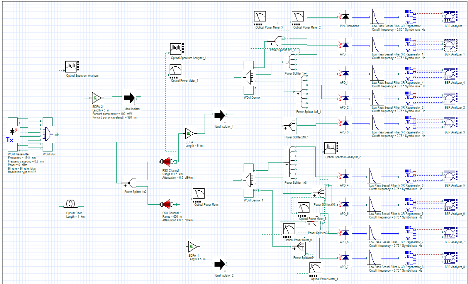
Şekil 1. Tasarlanan dalga boyu bölmeli hibrit optik haberleşme düzeneği
