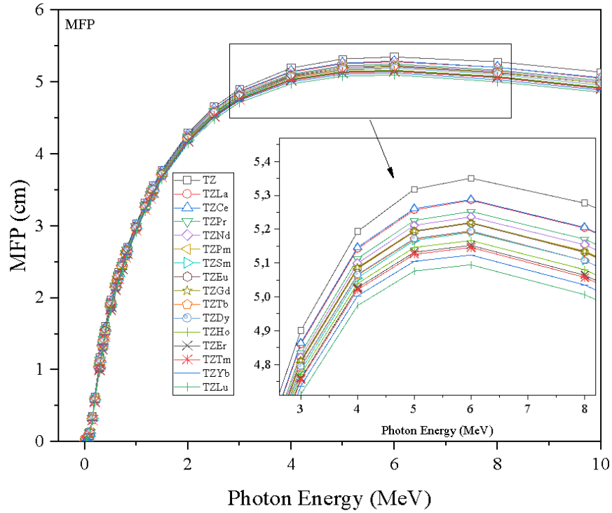
Şekil 4. Numunelere ait ortalama serbest yol ~ foton enerjisi (photon energy) (MFP) grafiği
