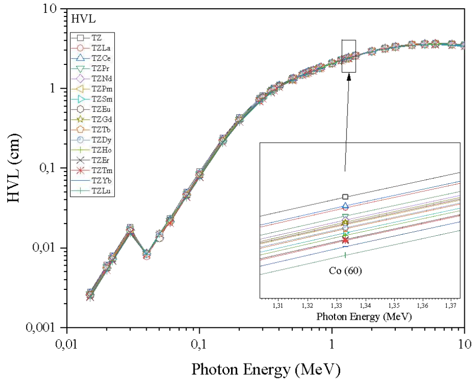
Şekil 3. Numunelere ait yarı değer katmanı ~ foton enerjisi (photon energy) (HVL) grafiği
