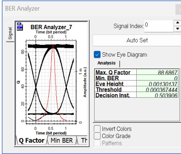
c) 5 Gbps, 600 m ve 32 kullanıcı
