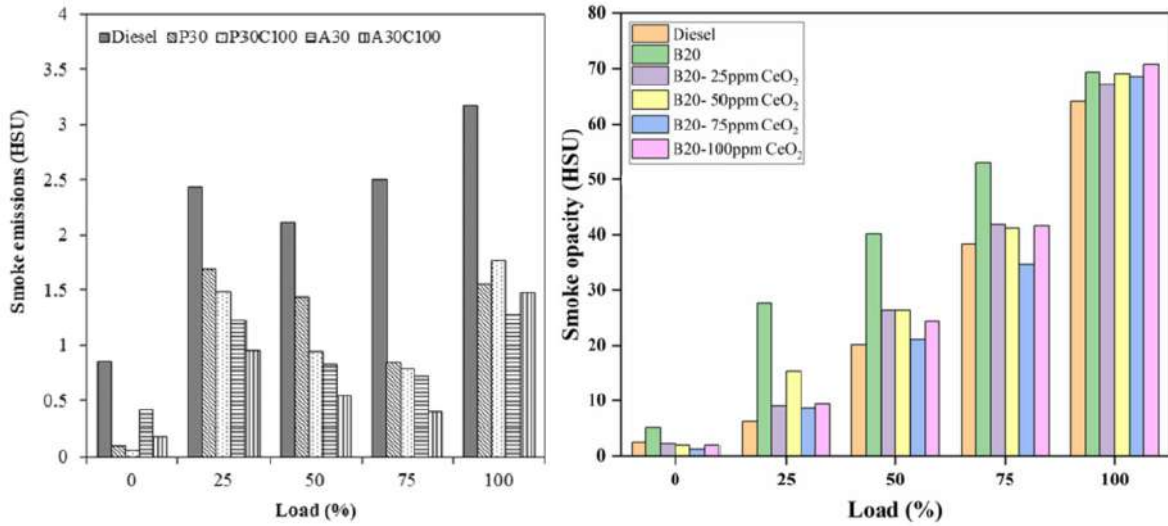
Şekil 9. Duman emisyonunun motor yüküne bağlı değişimi [3,5]
