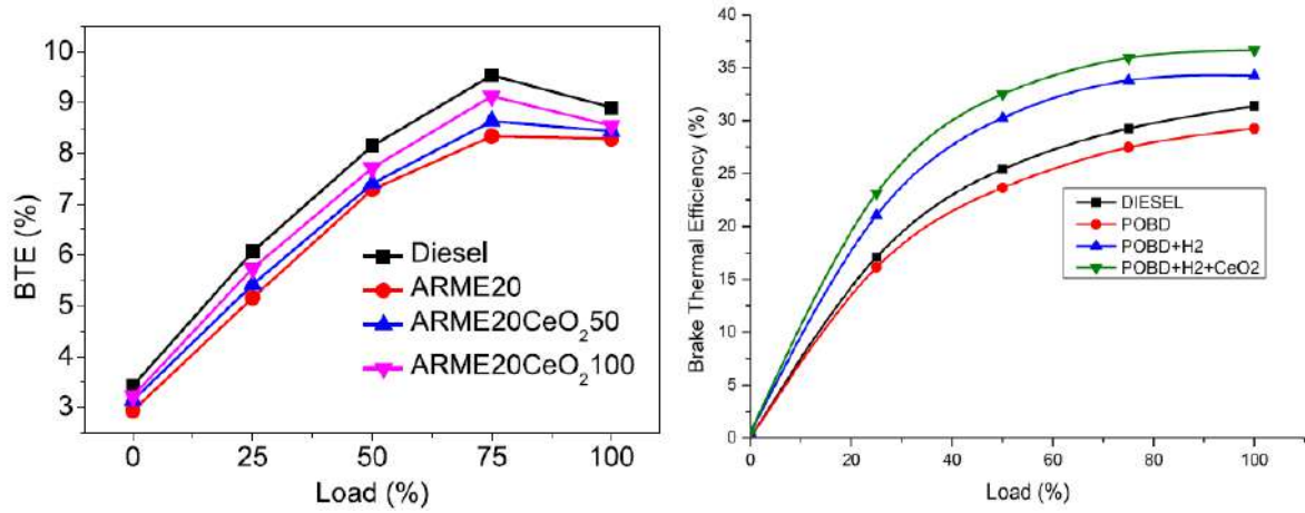
Şekil 4. Motor yüküne bağlı BTE değişimi [3,5,23,24]
