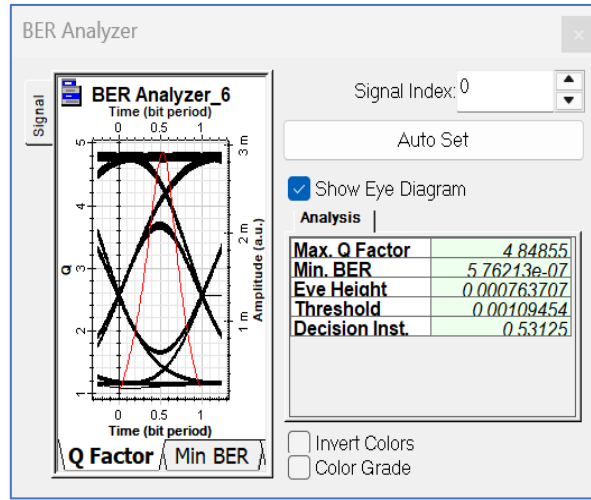
b) 10 Gbps, 600 m ve 16 kullanıcı
