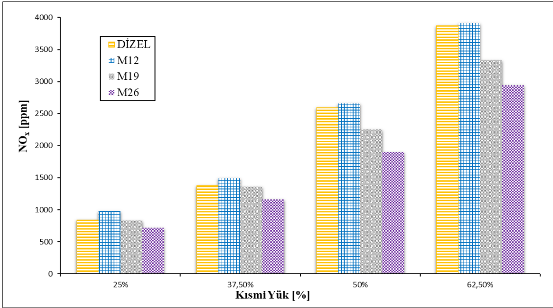
Şekil 11. Farklı kısmi yüklerde meydana gelen azotoksit emisyonlarının değişimi.
