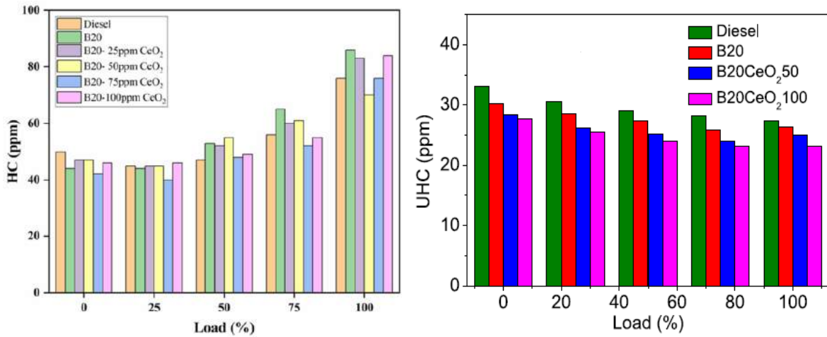
Şekil 7. HC emisyonunun motor yüküne bağlı değişimi[3,24]
