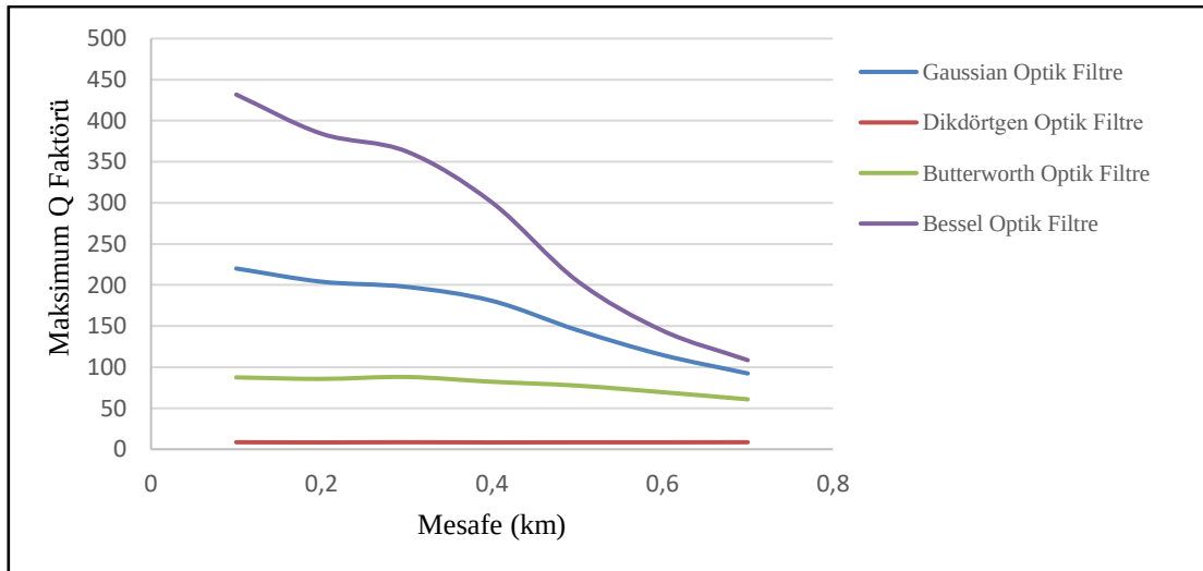
Şekil 6. Maksimum Q faktörünün mesafeye göre değişimi
