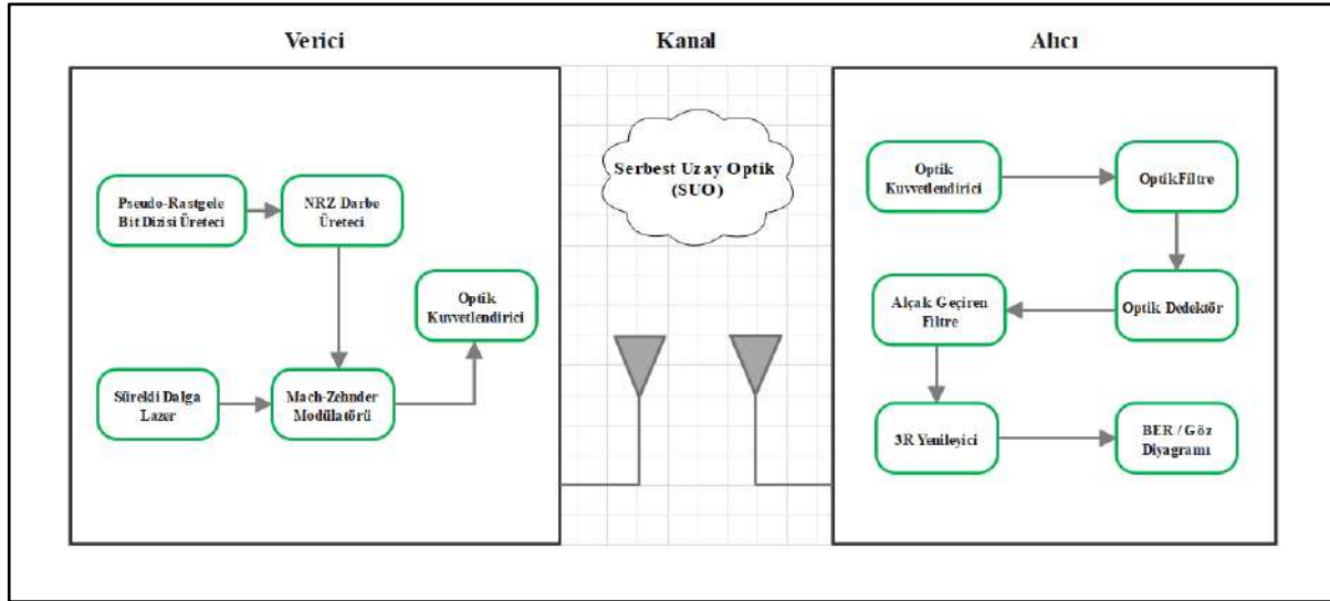
Şekil 1. Sistem modelinin blok diyagramı
