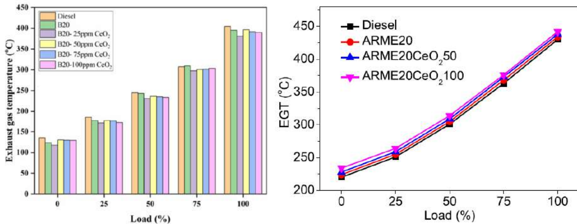
Şekil 6. Egzoz gaz sıcaklığının motor yüküne bağlı değişimi[3,24]
