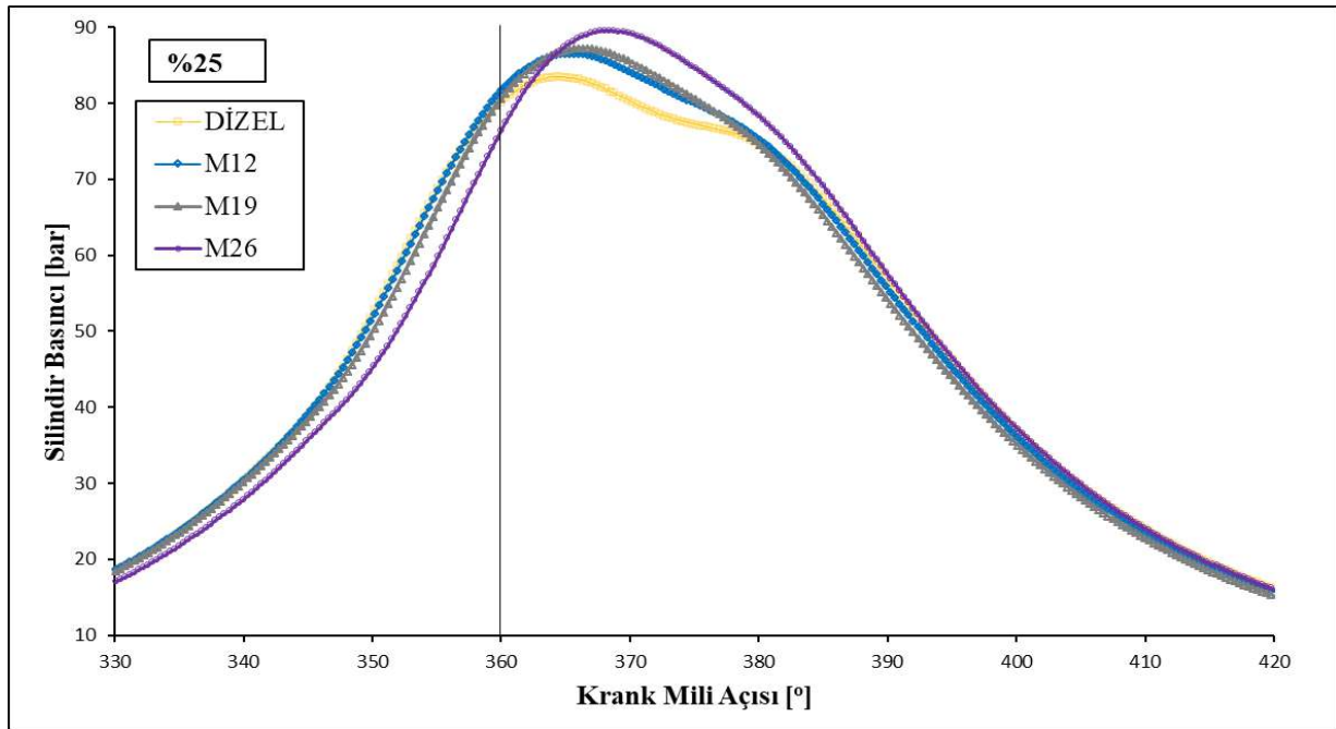
Şekil 2. %25 kısmi yükte dizel, M12, M19 ve M26 yakıtları için oluşan silindir basınçları
