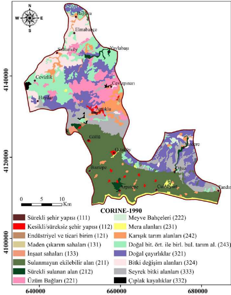
Şekil 3. 1990 yılına ait CORINE arazi örtüsü/kullanımı haritası
