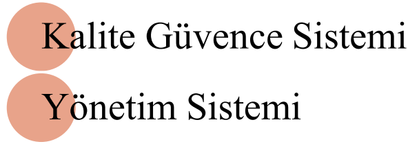
Şekil 3. Araştırma Temaları
