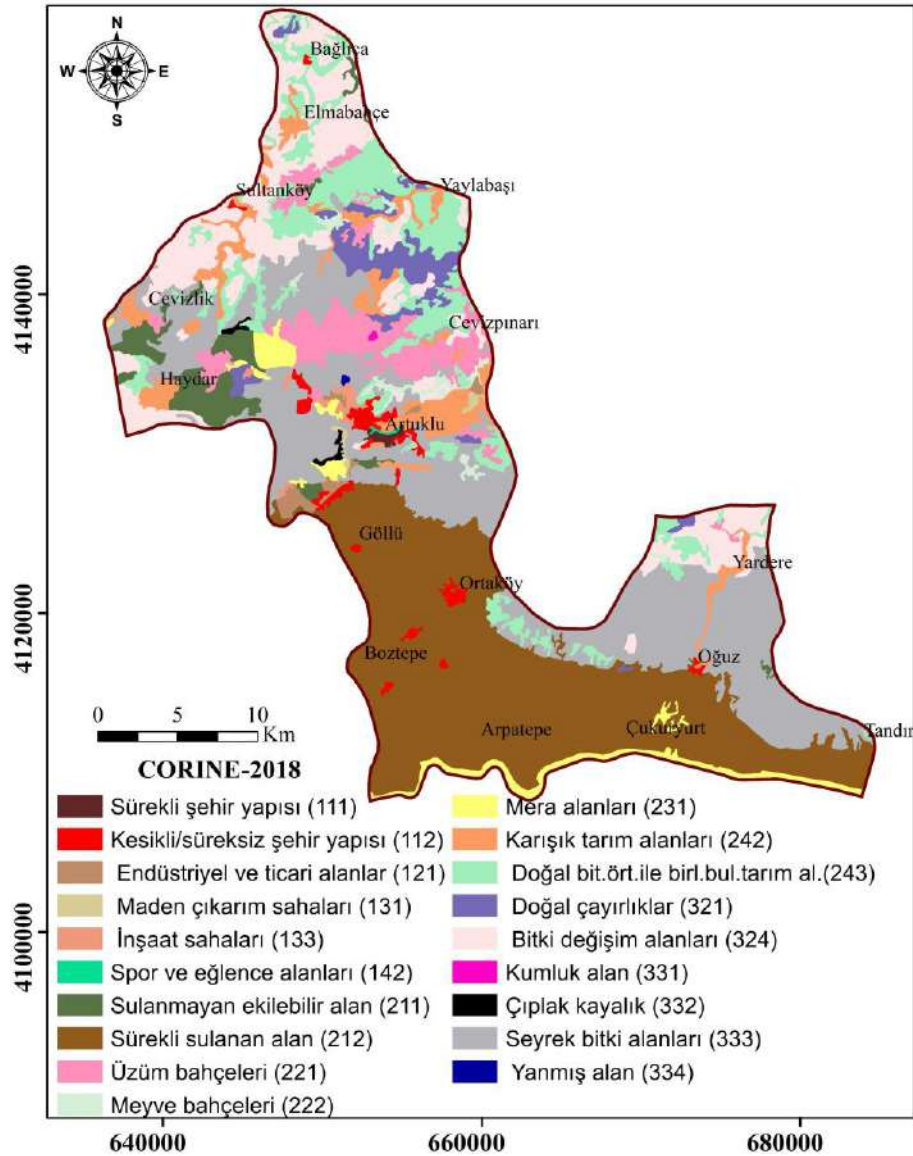
Şekil 7. 2018 yılına ait CORINE arazi örtüsü/kullanımı haritası
