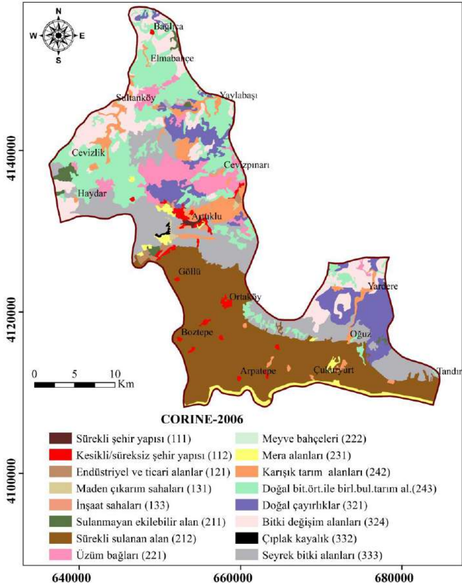
Şekil 5. 2006 yılına ait CORINE arazi örtüsü/kullanımı haritası
