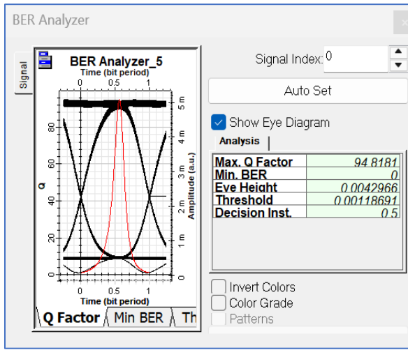
a) 5 Gbps, 600 m ve 8 kullanıcı
