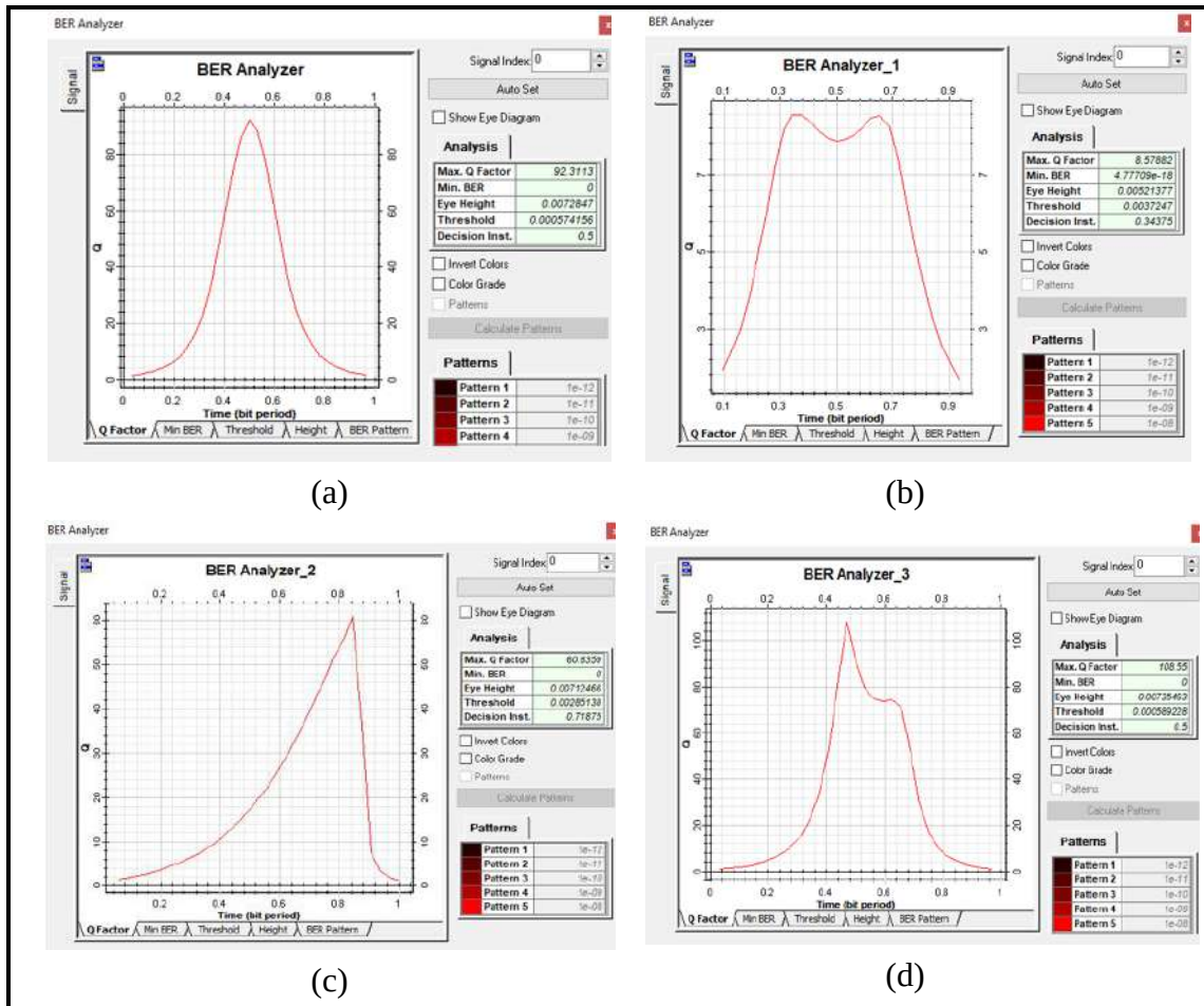
Şekil 5. (a) Gaussian optik filtre, (b) Dikdörtgen optik filtre, (c) Butterworth optik filtre ve (d) Bessel optik filtre için BER analizleri
