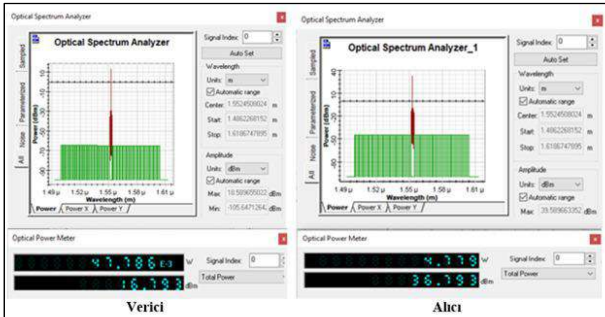
Şekil 4. Verici ve alıcı için optik spektrum analizör ve güç ölçer sonuçları
