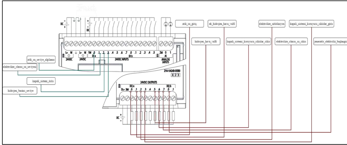
Şekil 1. PLC Giriş ve Çıkış Bağlantılarının Cihaza Entegrasyonu
